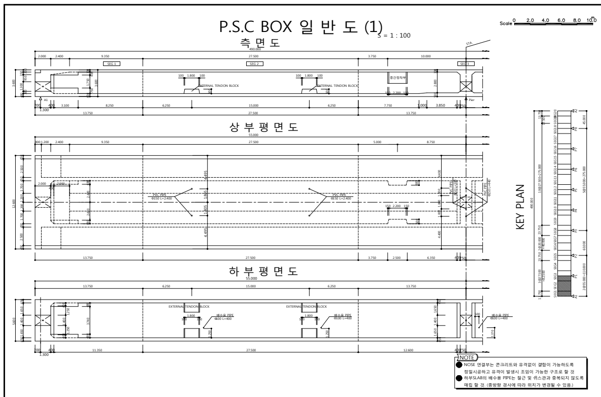
【그림 1.6】 발산1교(양양) P.S.C BOX 일반도
