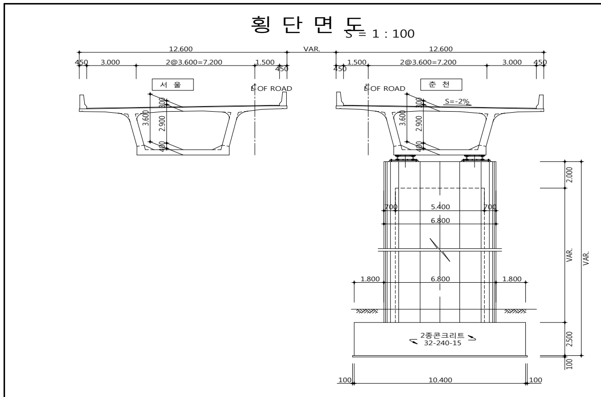
【그림 1.3】 발산1교(양양) 횡단면도
